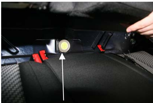
Abbildung 1: Crash Recorder
